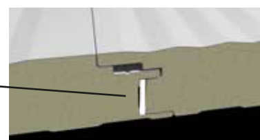
Dettaglio giunto - Joint Detail
